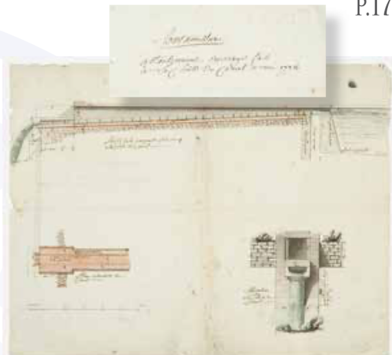
Un plan, une coupe et une élévation du nouvel exutoire du canal intitulé : Attachement ouvrages faits à la Chute du canal année 1778.
