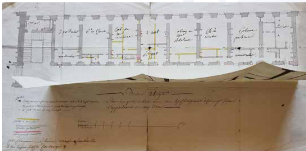
Plan avec retombe de la partie orientale du premier étage de l'aile Louis XV daté de 1783, intitulé : Plan de l'aile neuve avec les changements à faire p[ou]r former l'appartement de Mes Dames.
